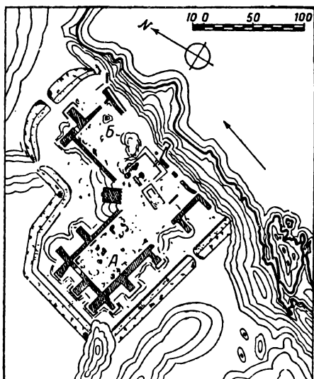
План египетской крепости в Семнэ
