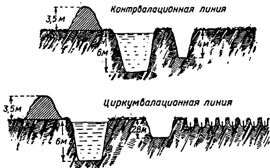
Осадные сооружения римлян под Алезией
